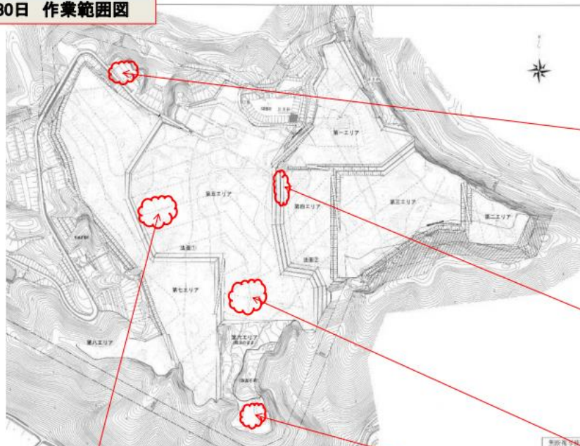
第5エリア 土工(掘削・盛土)
